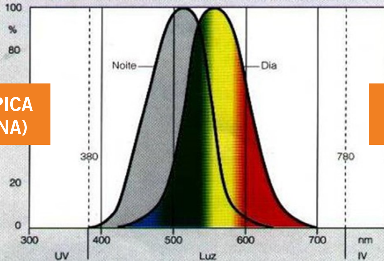
Fig. 2: Curva de sensibilidade do olho a radiações monocromáticas.
